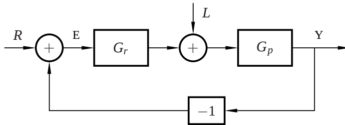
Figur 6 Blockschemat för slutna systemet vid reglering av övre tanken
