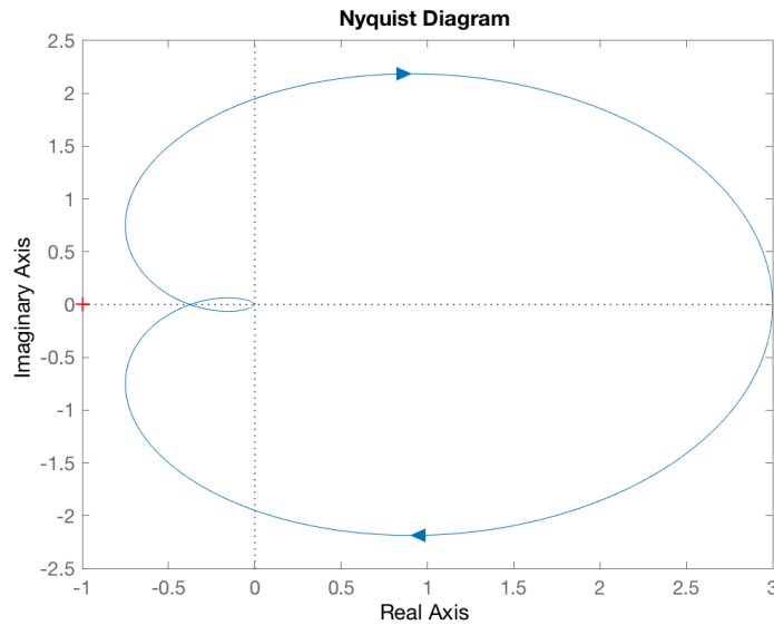
Figur 1 Nyquist-kurvan i 4.
